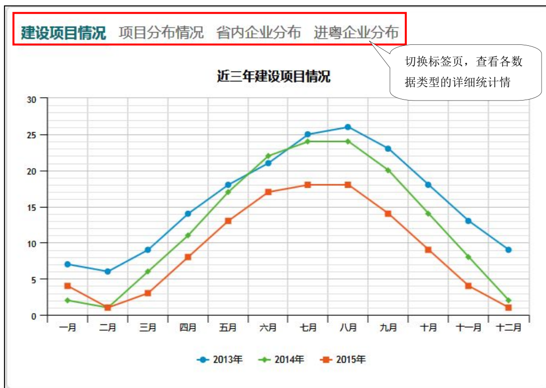
图 2.3.1 数据统计 1
