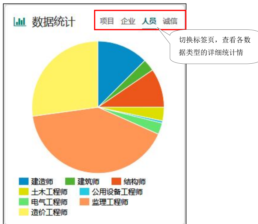
图 2.3.2 数据统计 2
