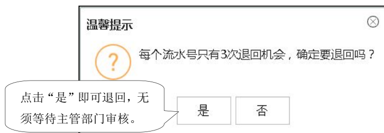
图 3.6.8 退回申请
