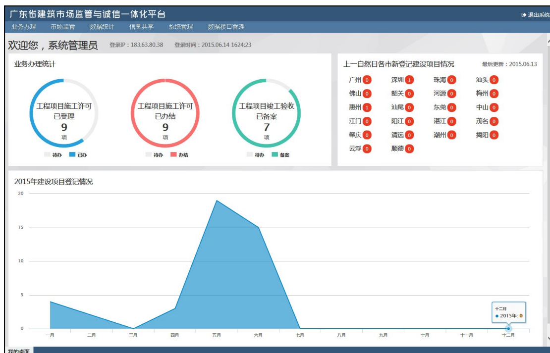
图 4.1.2 我的桌面
